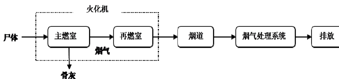
图 11 遗体火化火化工艺示意图
