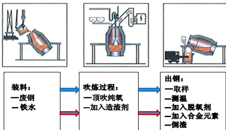
图 5 氧气顶吹转炉炼钢操作过程
